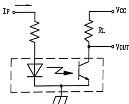
应答时间测试电路 Switch Time Test Circuit
